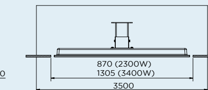
MINIMALE INBOUWRUIMTE OPTIE 2
