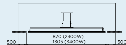
MINIMALE INBOUWRUIMTE OPTIE 1
